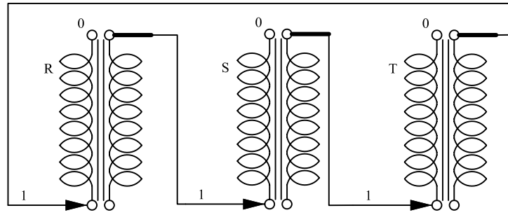
TRİSTÖR CİHAZLARININ STANDART ÜÇGEN BAĞLANTI ŞEKLİ
