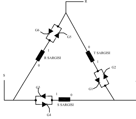
TRİSTÖRLERİN R-S-T BAĞLANTI DİYAGRAMI
