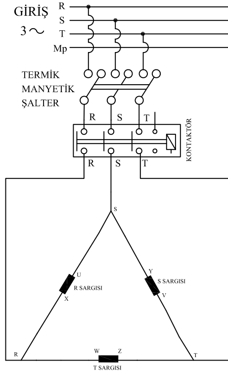
R-S-T BAĞLANTI DİYAGRAMI
