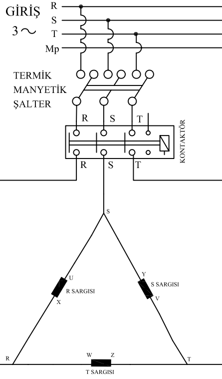
R-S-T BAĞLANTI DİYAGRAMI
