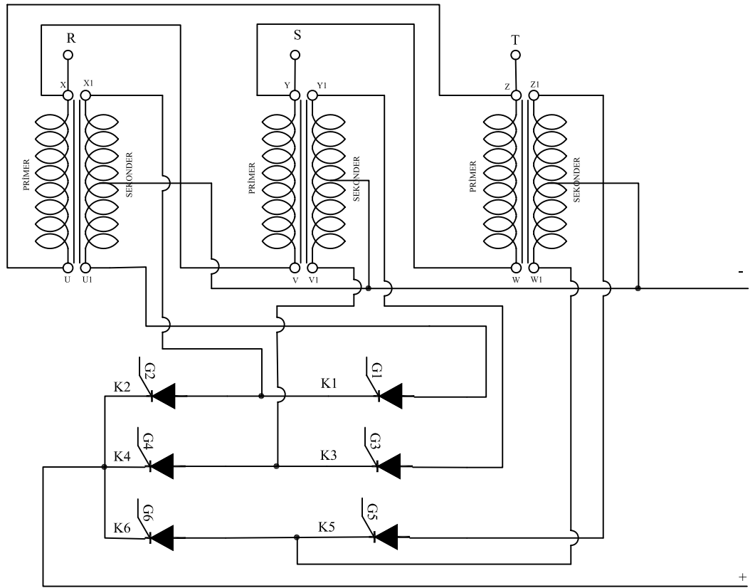
R-S-T BAĞLANTI DİYAGRAMI
