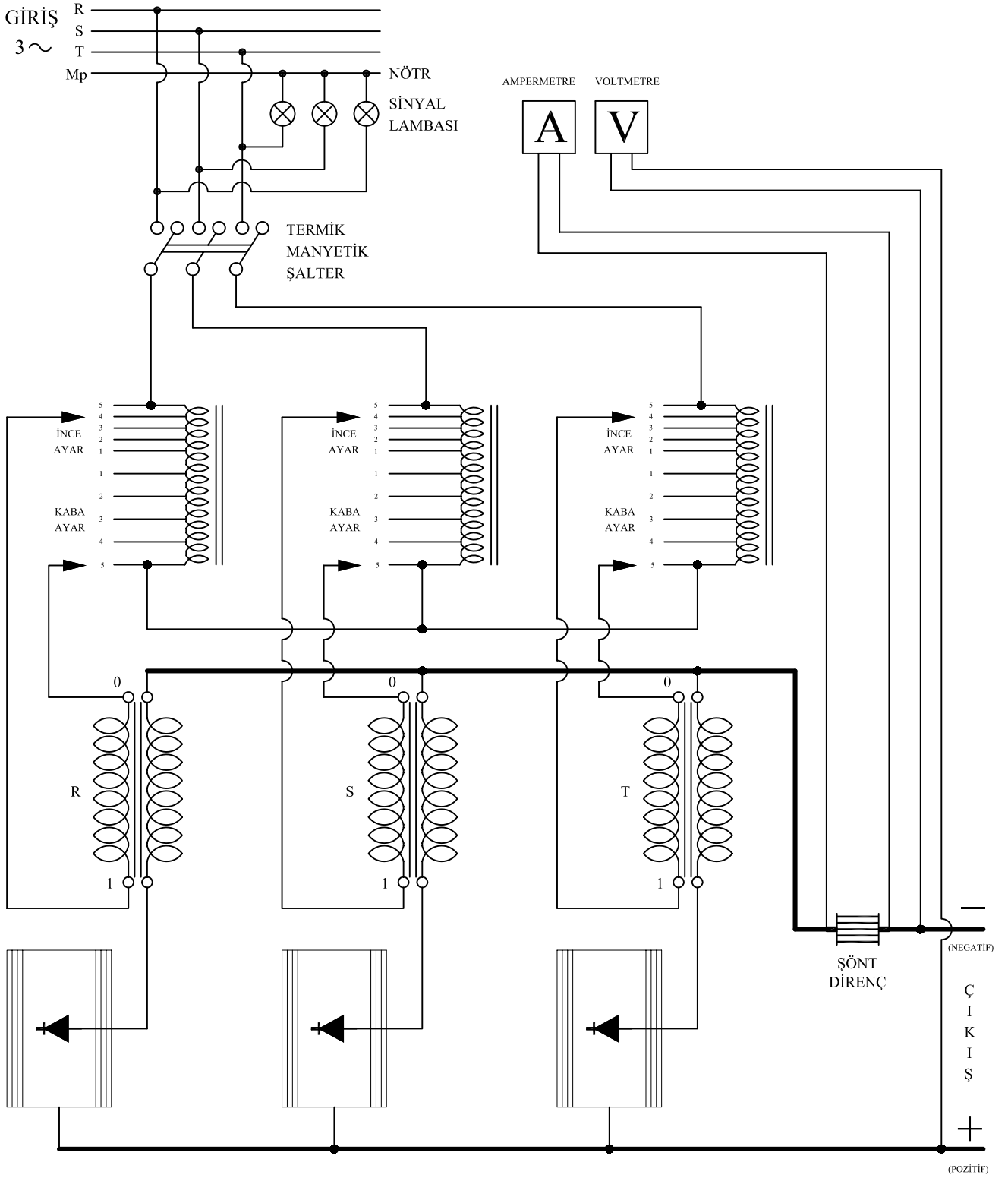
DİYOTLARIN BAĞLANTI ŞEKLİ : DS
